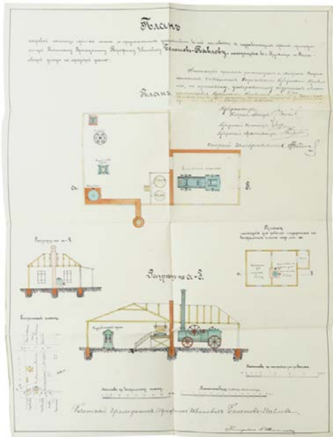
746 [Пешков, Н.Н., автограф] План паровой мельницы простого помола с предполагаемым устройством в ней маслобойни с гидравлическим прессом, принадлежащей почет. граждан. Т.И. Большов-Павлову.
