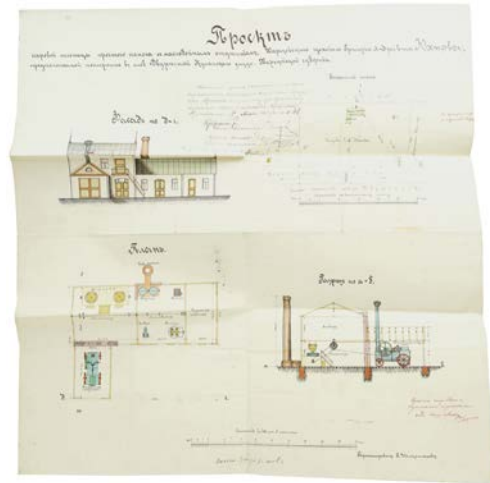
747 [Пешков, Н.Н., автограф] Проект паровой мельницы простого помола с маслобойным отделением / Проектировал Г. Шелкоплясов.
